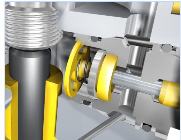
Einlassventilbaugruppe einer 200-Bar-Benzin-Einspritzpumpe.
